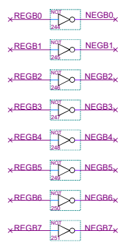
Negate B
