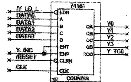
Y Index Register
