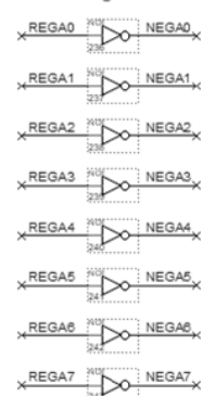
Negate A
