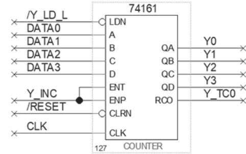
Y Index Register
