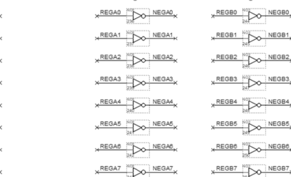
Negate A
